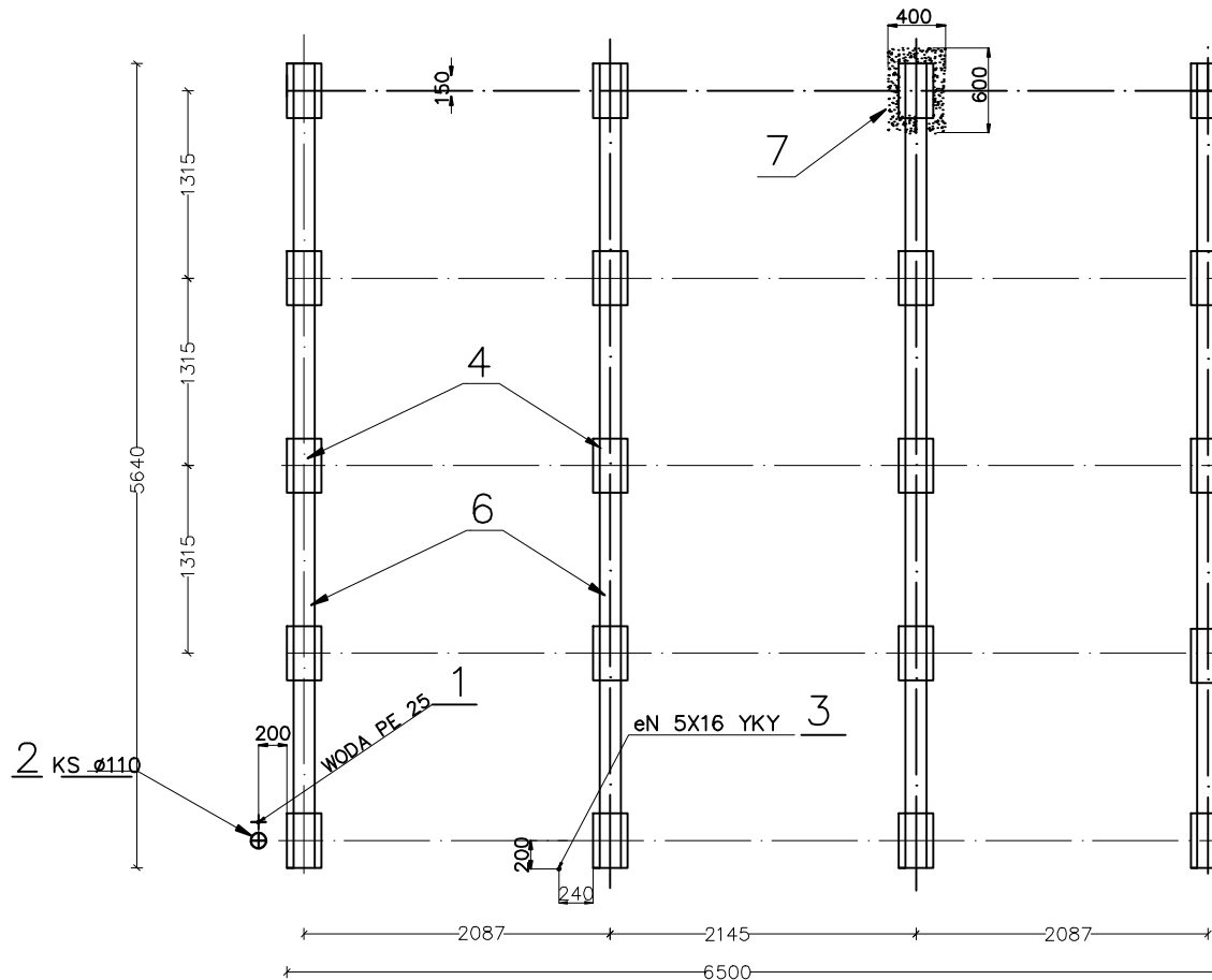
UKŁAD FUNDAMENTOWY POD PRZENOSNY BUDYNEK SOCJALNY O POW. 2 33M
