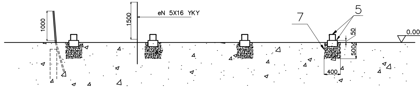
UKŁAD FUNDAMENTOWY POD PRZENOSNY BUDYNEK SOCJALNY O POW. 2 33M
